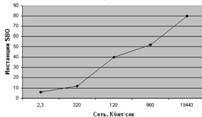
Загрузка сети по отношению к количеству запущенных инстанций SBO
