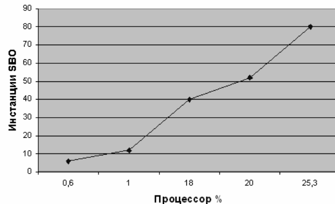
Загрузка ЦП по отношению к количеству запущенных инстанций SBO
