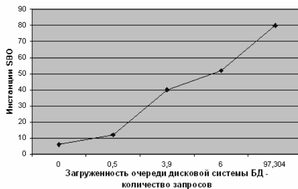
Загрузка очереди дисковой системы БД по отношению к количеству запущенных инстанций SBO
